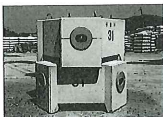
タコ産卵礁 (オクトム)
